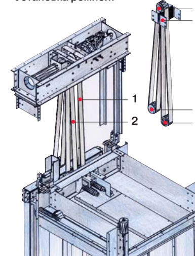
1. Ремень 1. 2. Ремень 2. 3. КВШ. 4. Шкив противовеса. 5. Шкив ремней кабины. 6. Пластина крепления
