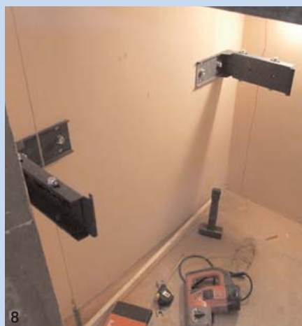
8. Установка направляющих требует предельной точности. Их монтируют, используя отвесы
